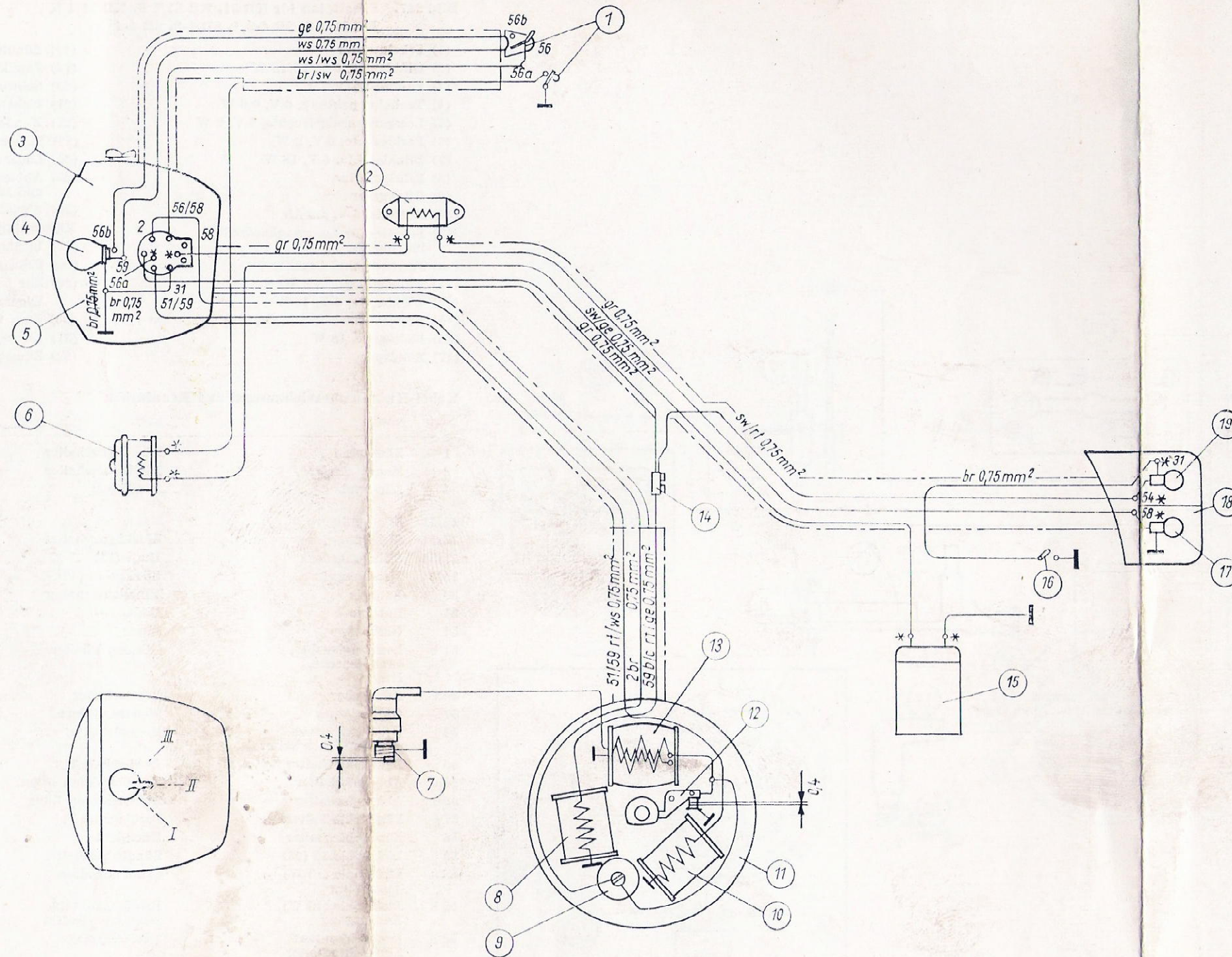
Bild 246. Schaltplan
