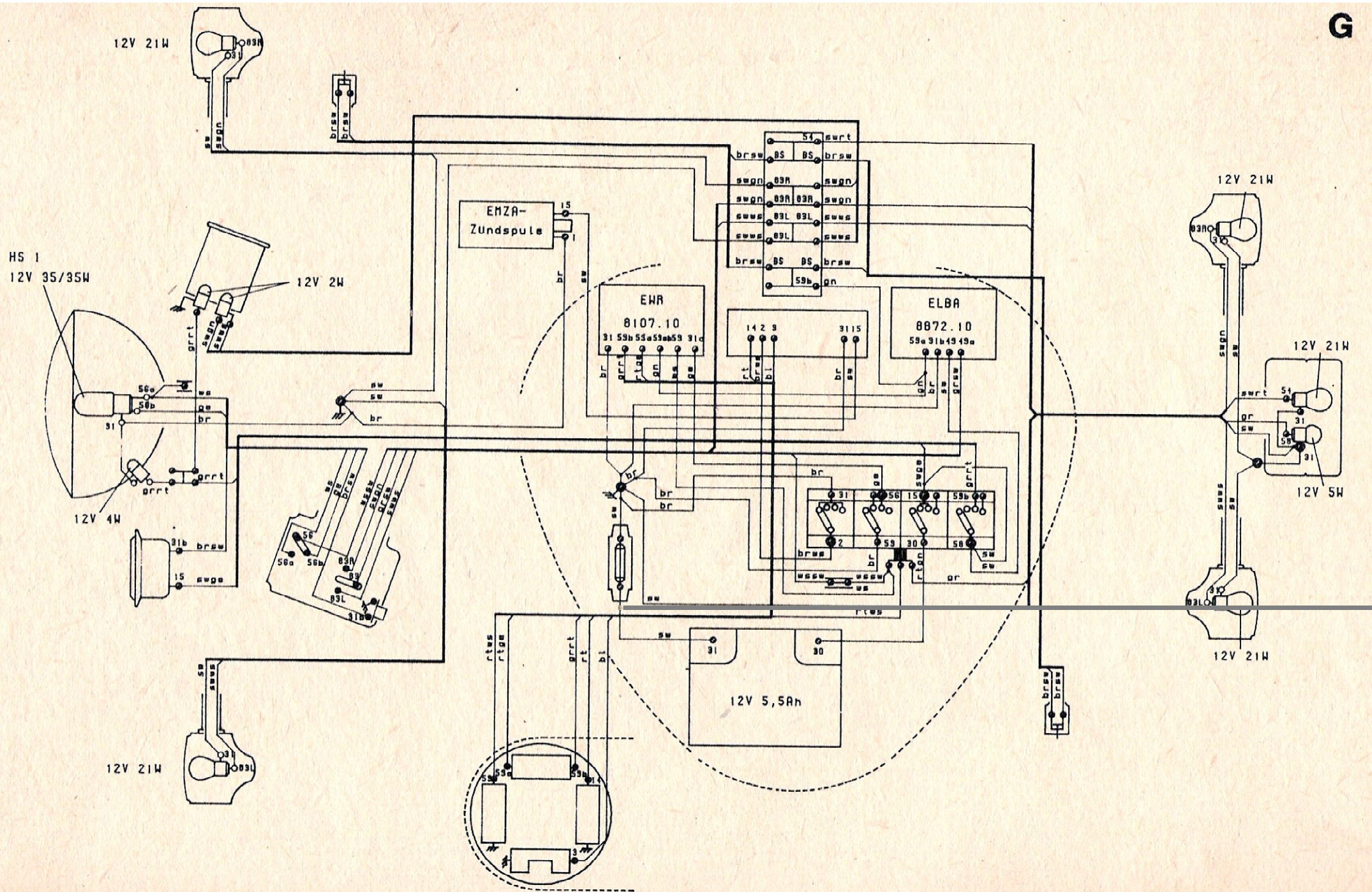
Bild 220. Schaltplan für S 51/1 C 1, S 51/1 E S 51/1 E 1 und S 70/1 E
